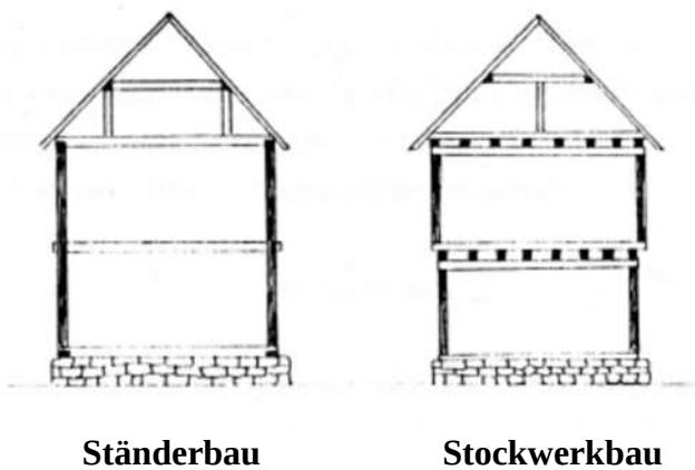
Abb 3: Fachwerkhaus-Grundtypen
